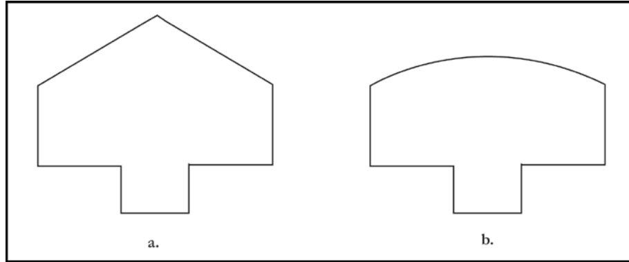
Resim 4: a. Semerdam, beşik çatılı oda mezar çizimi, b. Tonoz çatılı oda mezar çizimi.
