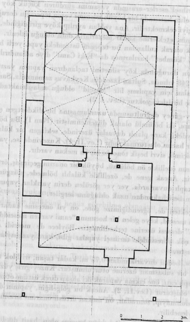
PLAN I - MÜLK KOYU - TÜRBELİ MESCİDİ PLANI 0:1/50
