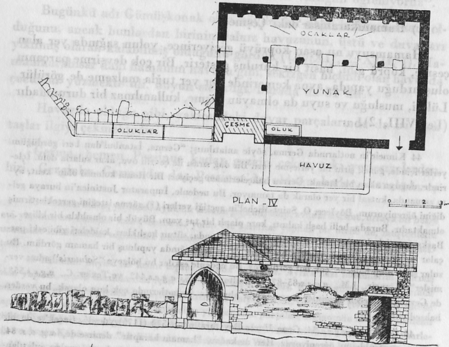
ŞEKİL 7 YUNAK ve ÇEŞMENİN ÖNDEN GÖRÜŞÜ
