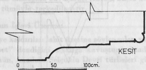
ŞEKİL-2 MÜLK KÖYÜ - TÜRBELİ MESCİT İÇ KAPI AYRINTISI Ö:1/20
