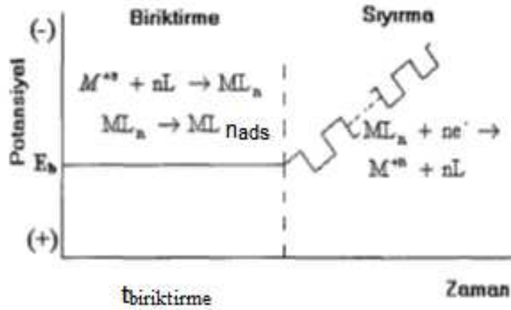
Şekil 2.14 Adsorptif sıyırma voltametrisinin şematik gösterimi
