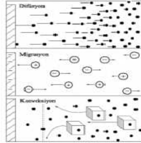
Şekil 2.4 Elektrot üzerinde kütle aktarımı gösterimi
