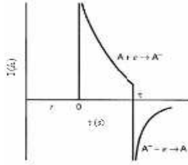
Şekil 2.16 Kronoamperometride akım-zaman ilişkisi
