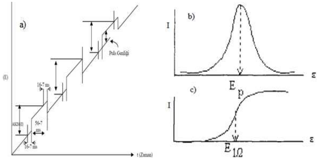
Şekil 2.10.a.DPV'de uygulanan potansiyelin zaman ile deęişimi, b.DPV'de akım potansiyel eęrisi. c.DA'da akım-potansiyel eęrisi
