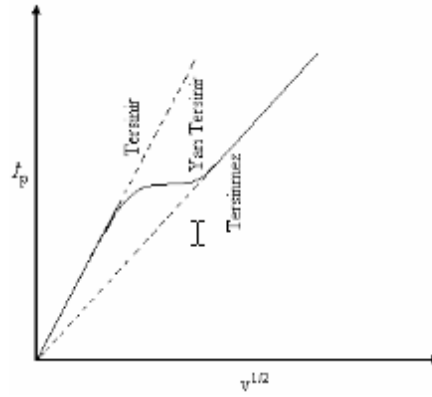
Şekil 2.9 Dönüşümlü voltametrde pik akımının tarama hızının karekökü ile değişimi
