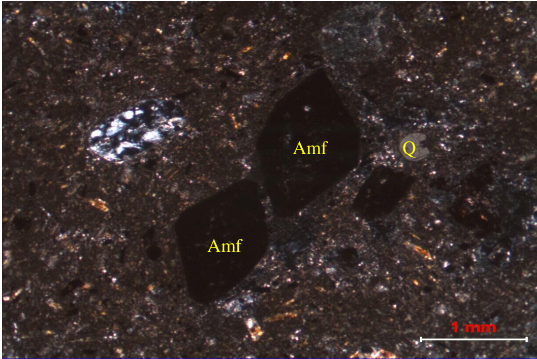
Foto 2.12 Hiyalopilitik dokulu, opasitlemiş amfibol ve körfez dokusu gösteren kuvars içeren dasitin mikrofotografı (2.nikol) (Amf: Amfibol, Q: Kuvars)
