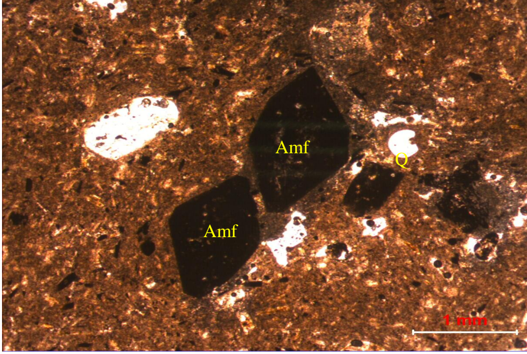
Foto 2.11 Hiyalopilitik dokulu, opasitlemiş amfibol ve körfez dokusu gösteren kuvars içeren dasitin mikrofotografı (1.nikol) (Amf: Amfibol, Q: Kuvars)
