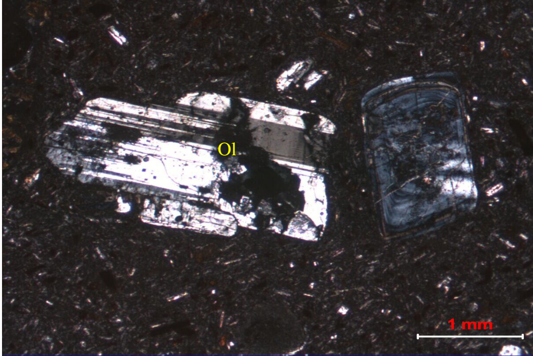
Foto 2.10 Hyalopilitik dokulu zonlanma gösteren oligoklaz içeren dasitin mikrofotografı (Ol: Oligoklaz)
