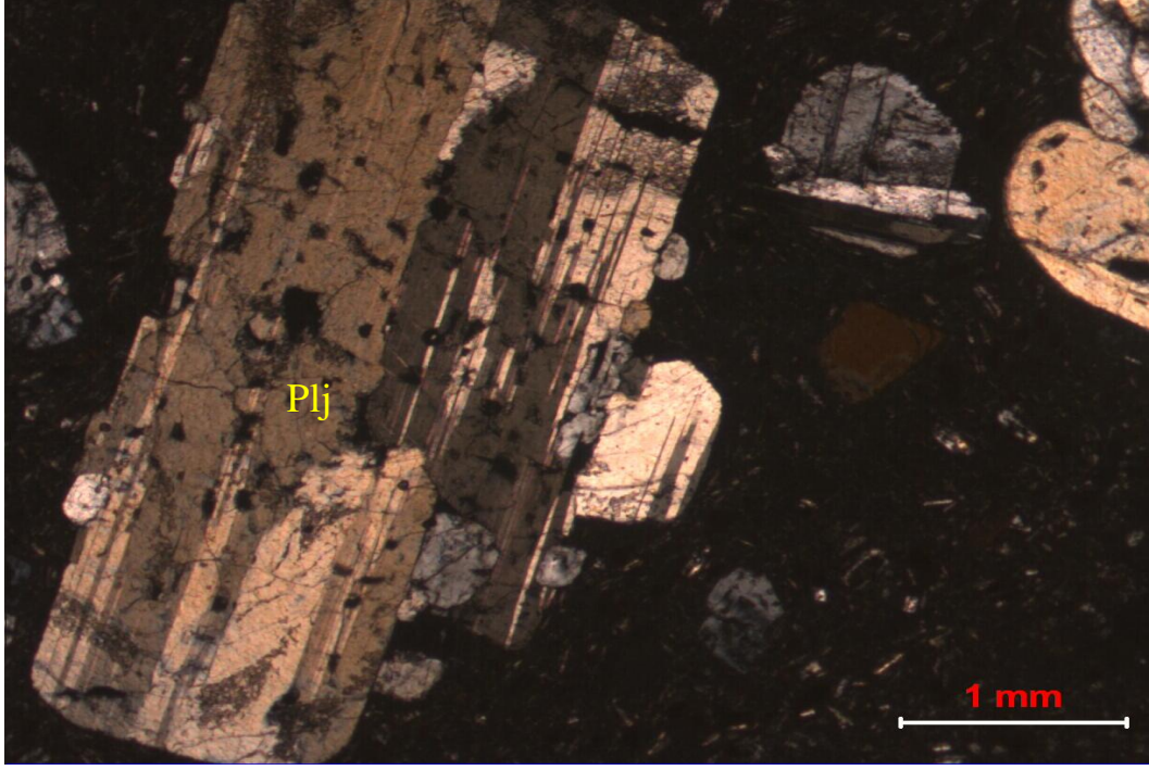
Foto 2.9 Hyalopilitik dokulu kum plajiyoklazdan oluşan dasitin mikrofotografı (Plj: Plajiyoklas)
