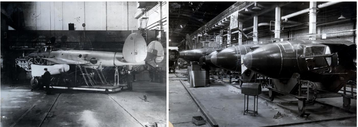
22 No'lu Fabrikada uçak yapımı ve montaj çalışmaları – S. P. Garbunov Uçak Fabrikası Müzesi- Kazan
