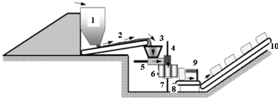
Şekil 1- Silaj paketleme tesisinin şematik gösterimi: 1, ürün deposu; 2, uzun taşıma elevatörü; 3, tartım ünitesi; 4, sıkıştırma kovanı; 5, itici hazne; 6, sıkıştırma kovanı; 7, hareketli alt destek platformu; 8, kısa taşıma elevatörü; 9, termik yapıştırma ünitesi; 10, yükleme elevatörü (Çakmak et al 2007)
