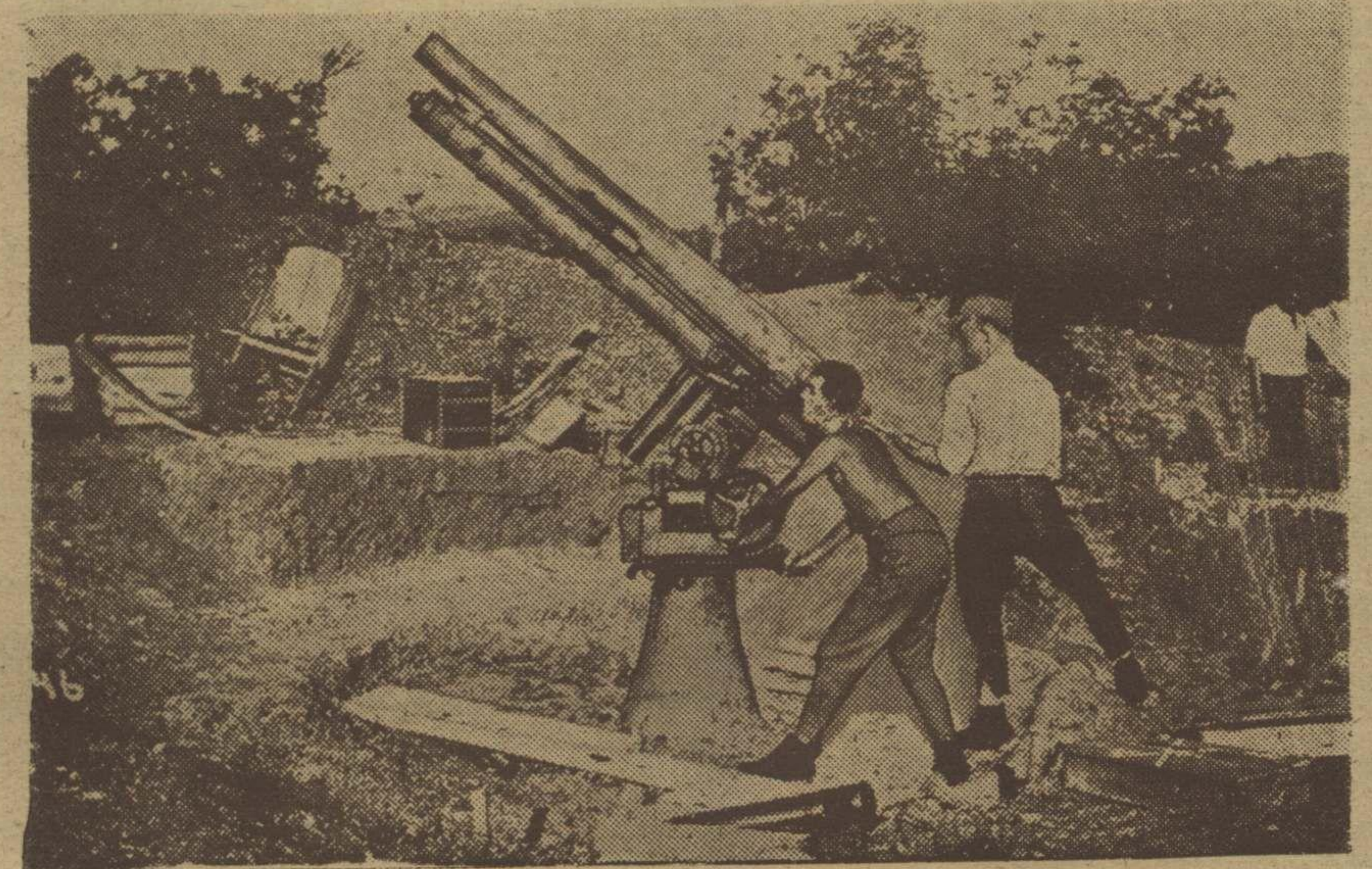
ایزوتزو جبهه سنده : آوستریا و مجارستان اردوسنك دشمن طیاره لرینه قارشى بر طوی، حال فعالیتده Poste anti-aérien austro-hongrois sur l'Isonzo.
