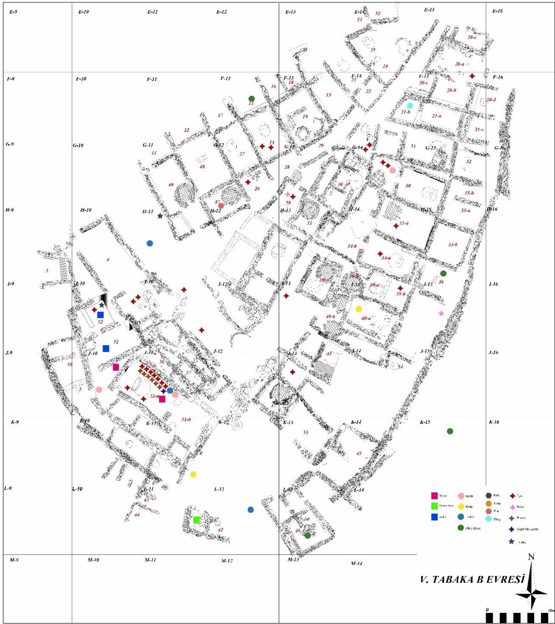
Plan 3: Seyitömer Höyük V. Tabaka B Evresi Yerleşim Planı Üzerinde Buluntuların Dağılımı
