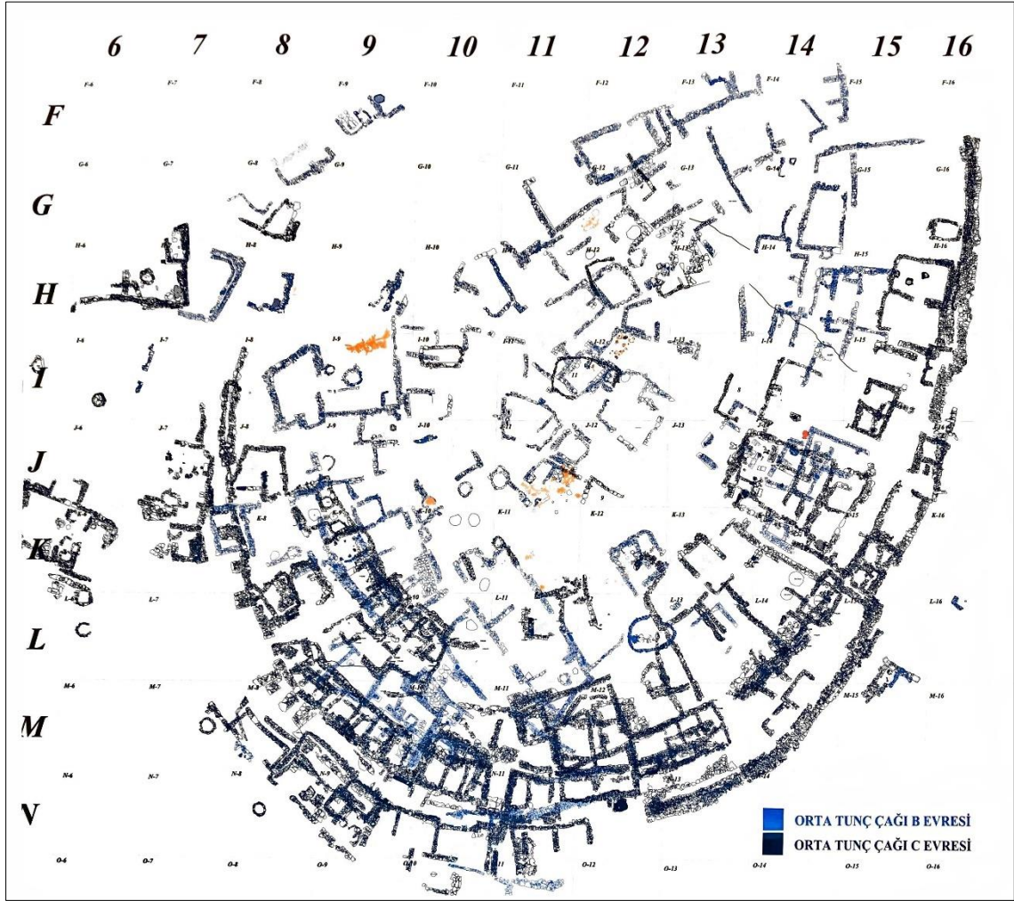
Plan 1: Seyitömer Höyük IV. Tabaka B ve C Evreleri Planı
