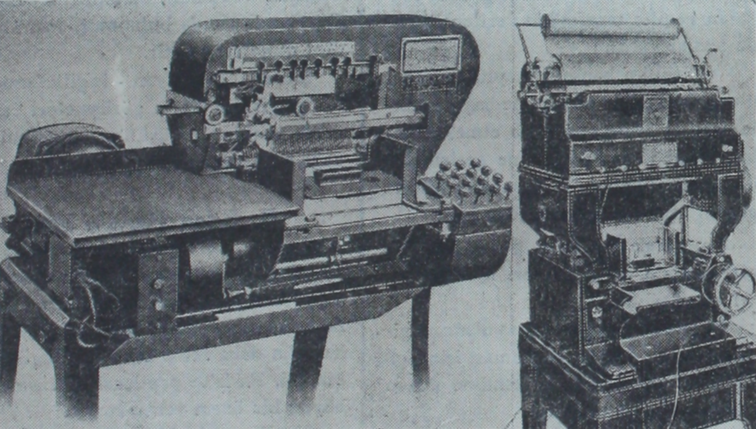
Bize sayımın sonuçlarını üç günde bildirecek olan İstatistik Genel Direktörlüğünün son sistem iki delme ve toplama makinası
