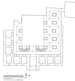
5- Bali Bey Hanı Zemin Kat Restitüsyonu (G. Yılmaz'dan değiştirilerek)
