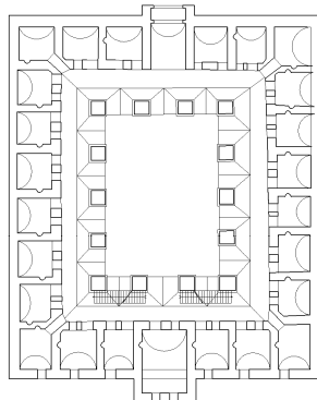
BURSA BALI BEY HANI RESTİTÜSYON ÜÇÜNCÜ KAT ÇİZİMİ (Yılmaz'ın Çizimi)
