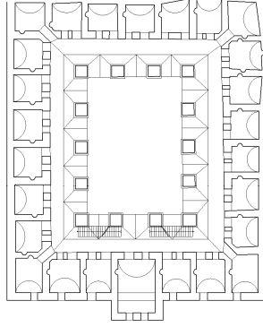
BURSA BALI BEY HANI RESTİTÜSYON BİRİNCİ KAT ÇİZİMİ (Yılmaz'ın Çizimi)
