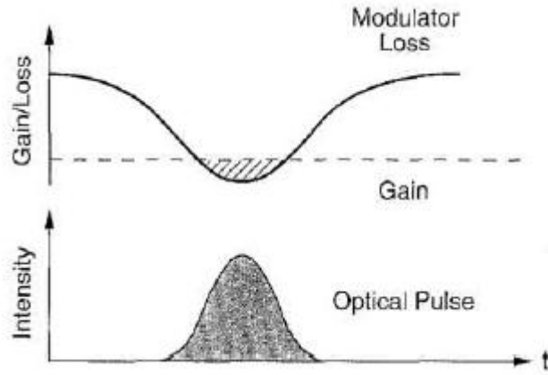
Şekil 2.8 Aktif Mod-Kilitleme Örneği
