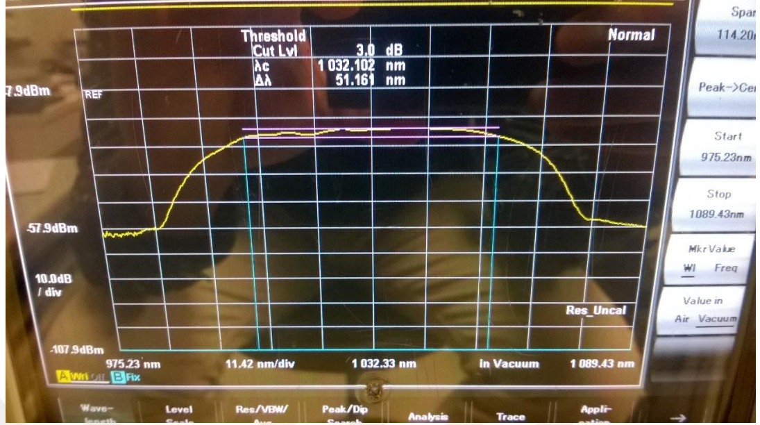
Şekil 4.2 Mod-kilitli bir hal bulunduktan sonra, lazerde oluşan atımların şekli
